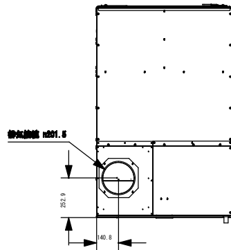
上面図
