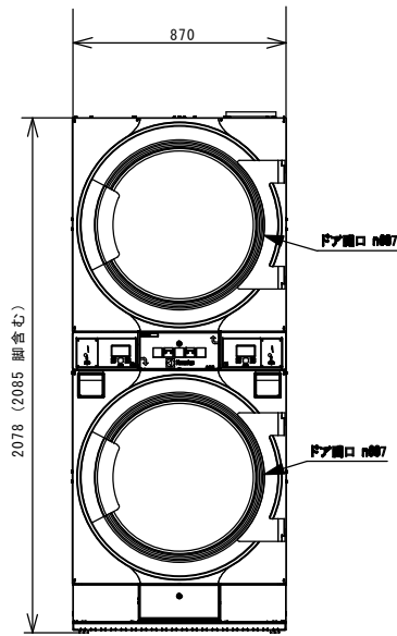
正面図
