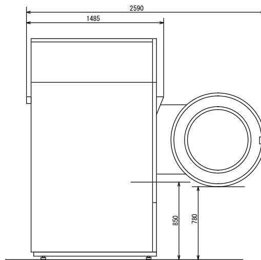
側面
