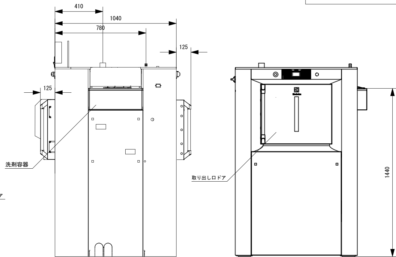
左側面図
