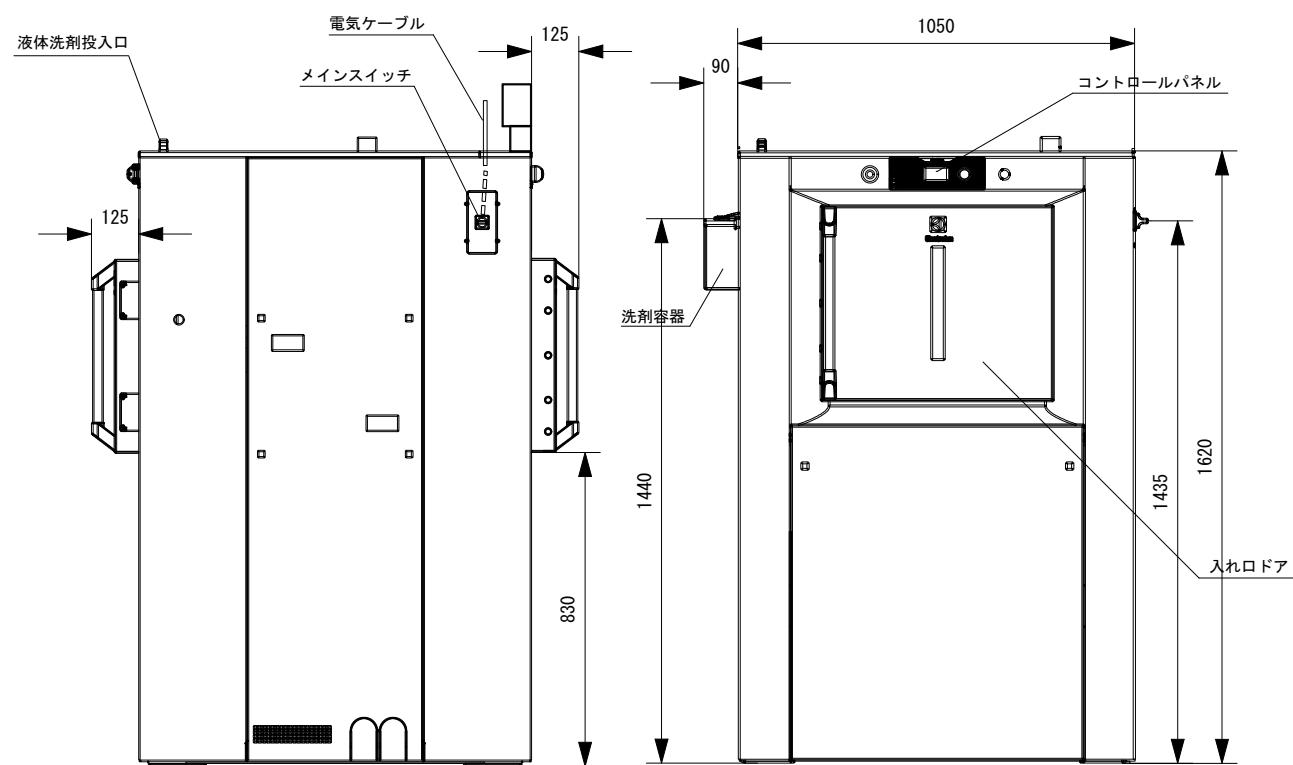
右側面図
