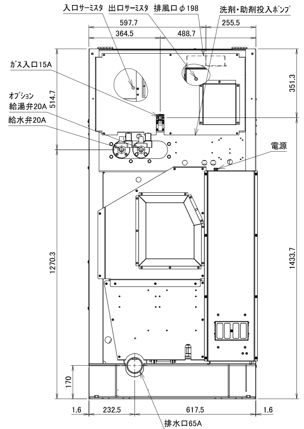
WD6-11JO2外観図
