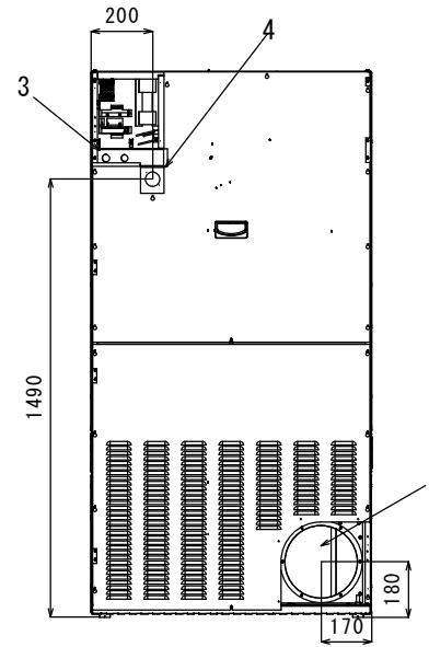
背面図
