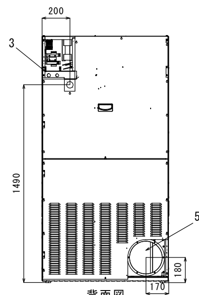
背面図
