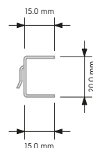
Sezione guida sinistra
