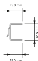
Sezione guida destra
