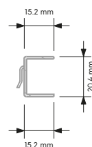
Sezione guida sinistra
