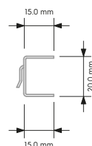
Sezione guida destra
